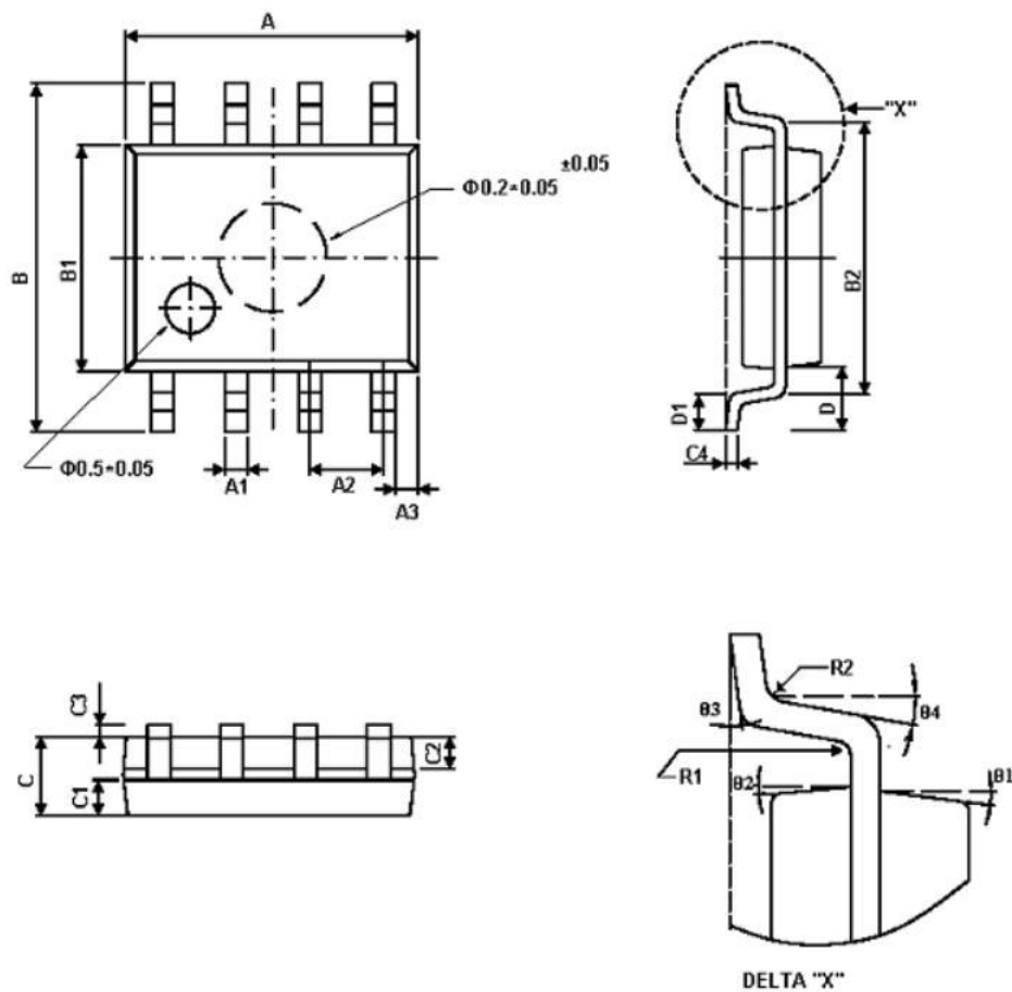
图11 芯片 SOP8封装尺寸信息
