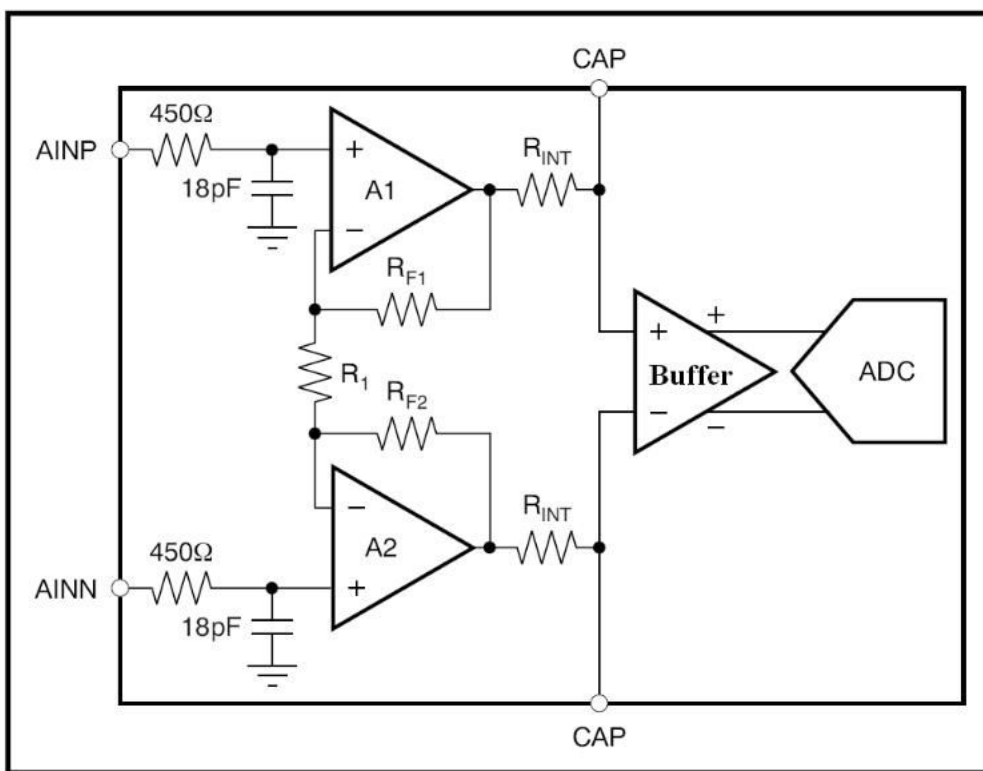
图4 PGA结构图
