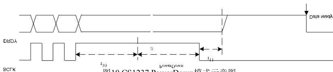
图10 CS1237 PowerDown模式示意图
