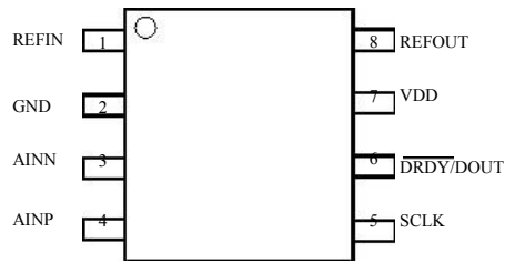
图2 CS1237芯片引脚图
