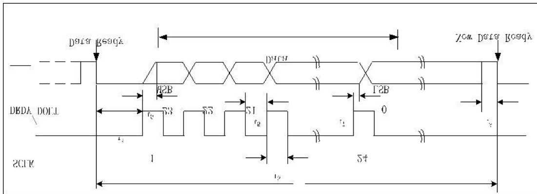
图7 CS1237读取数据时序图 1
